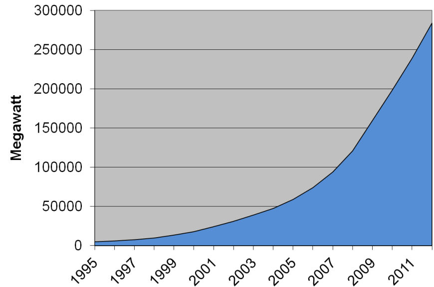
Weltweite Windenergie-Leistung in Megawatt (kumuliert)
