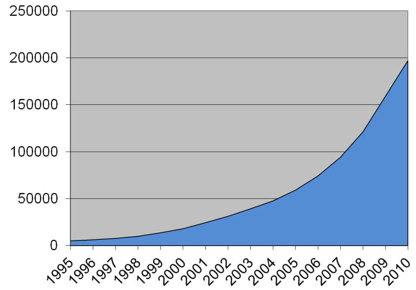
Weltweite Windenergie-Leistung in Megawatt (kumuliert)
